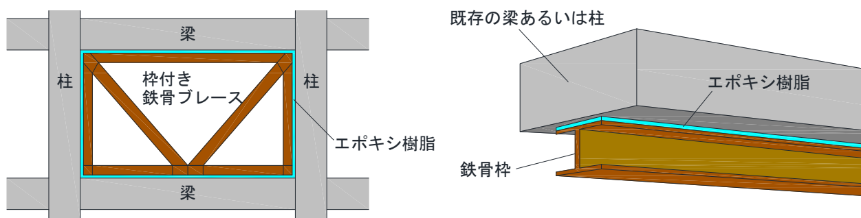
鉄骨ブレース接着工法の概要図
